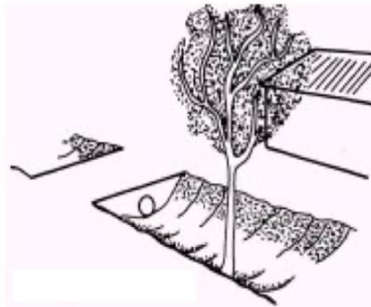
Exemple type d'une noue végétalisée
